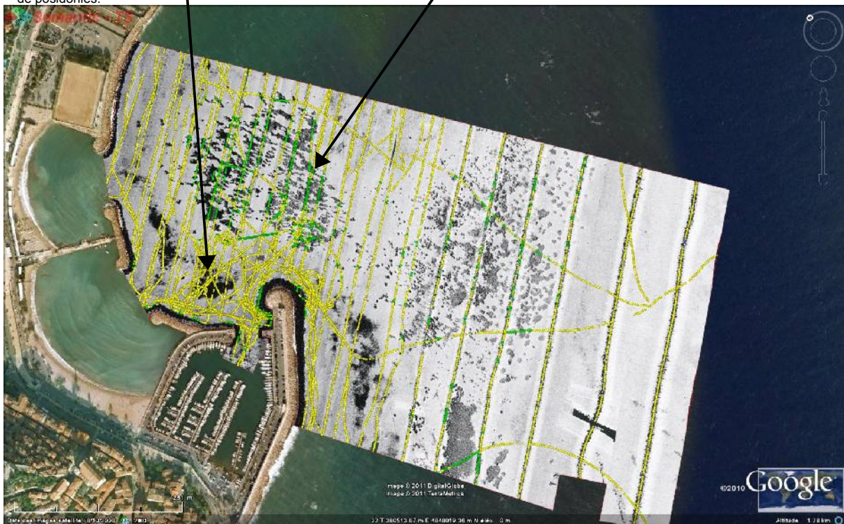
Figure 16: Mosaïque sonar latéral au large du port de Menton et SACLAF végétaux DIVA @SEMANTIC TS Apport du SACLAF DIVA pour l'aide à l'interprétation
