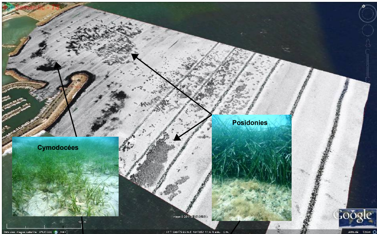
Figure 15: Mosaïque sonar latéral au large du port de Menton @SEMANTIC TS Observation de zone de forte réflectivité du fond. Observations sur le terrain : cymodocées et posidonies
