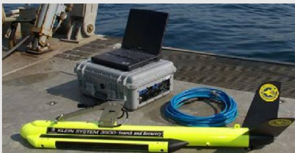
Sonar latéral tracté
