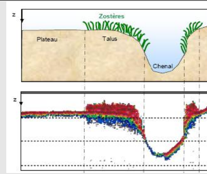
En haut : Schéma du milieu réel En bas : Réponse acoustique du sondeur
